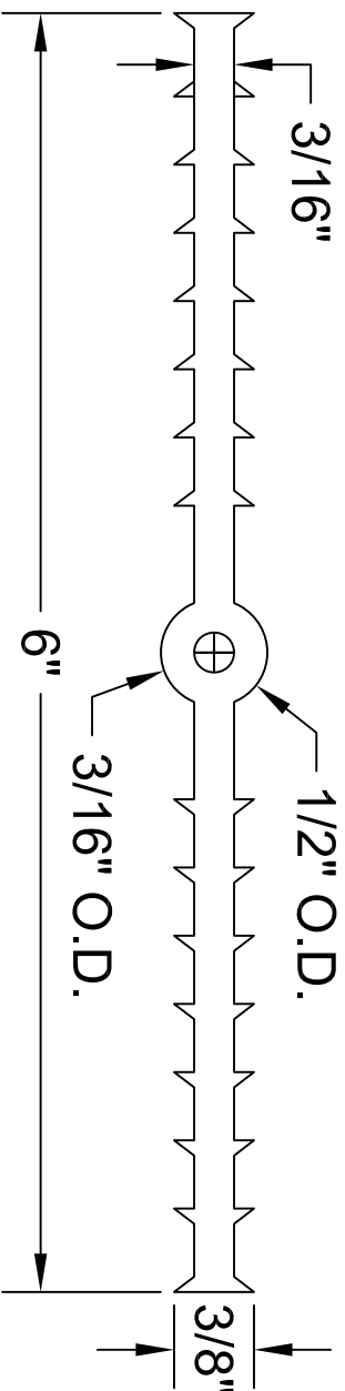
TCB-6316NT
